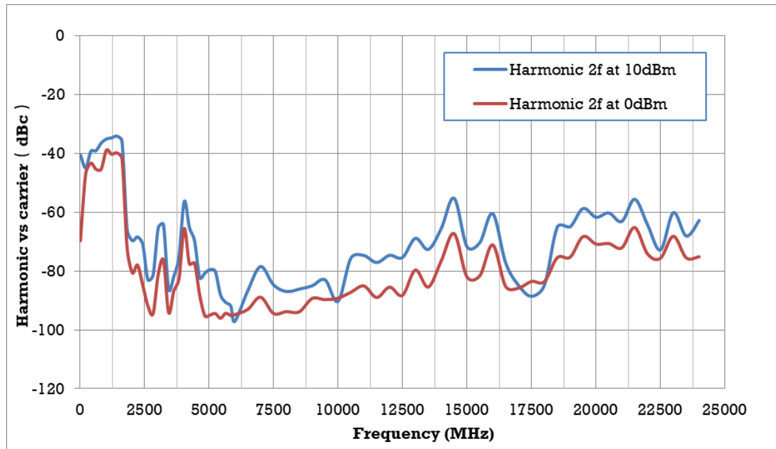
二次谐波 VS 载波频率, 输出电平=0 &amp; 10 dBm
