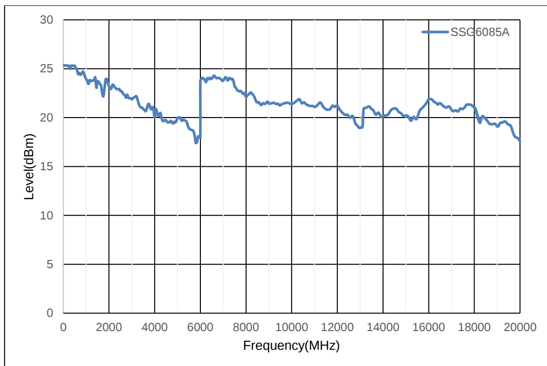
最大输出功率, SSG6085A (不保证指标精度)
