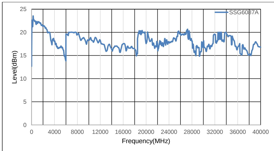
最大输出功率, SSG6087A (不保证指标精度)
