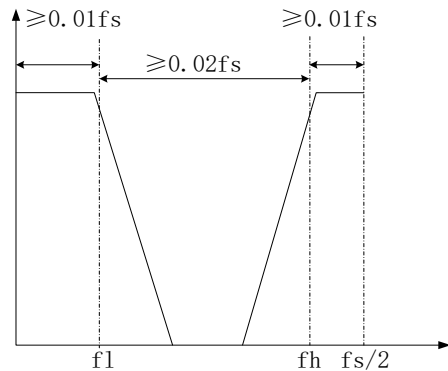
带阻
