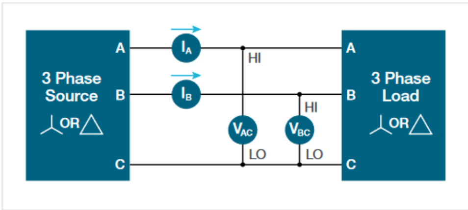
三相三线 (2V2I)
