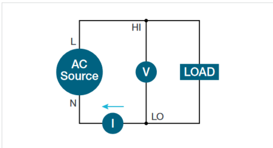
两相三线(2V2I)
