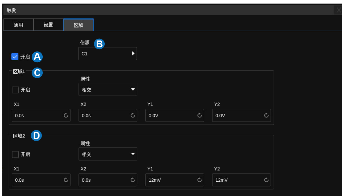
A. 开启/关闭区域触发
