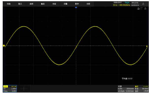
平均值模式 (32 倍)
