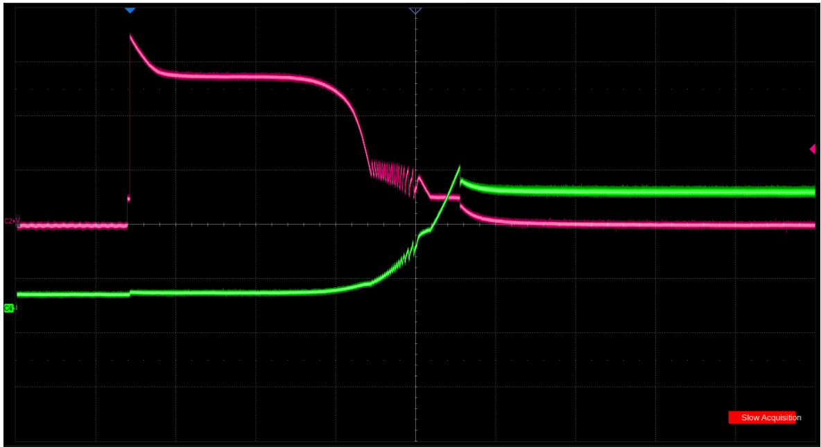
上电时 MOSFET 上的电压和电流波形
