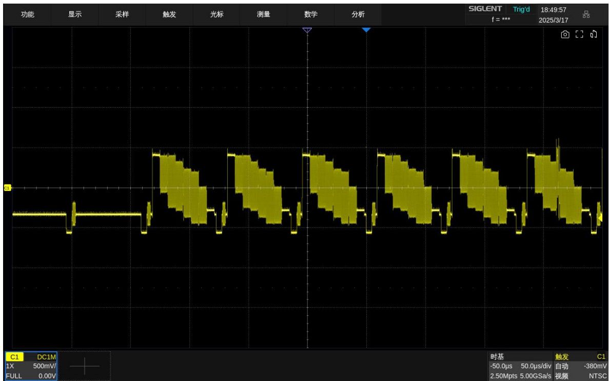
特定行上视频触发 (NTSC 标准)
