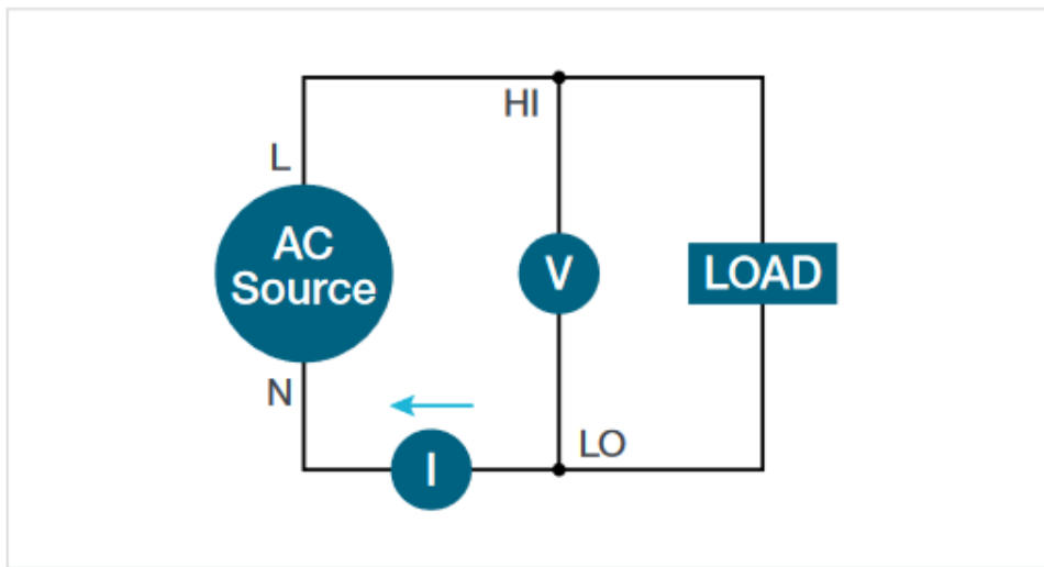
单相两线(1V1I)
