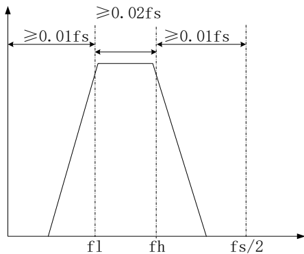
带通
