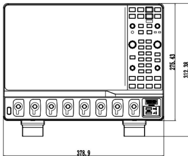
正视图
