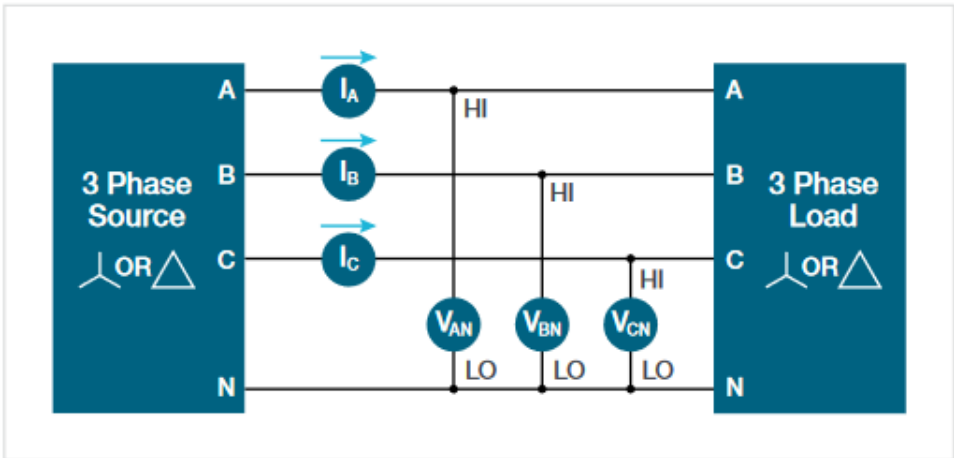
三相四线 (3V3I)
