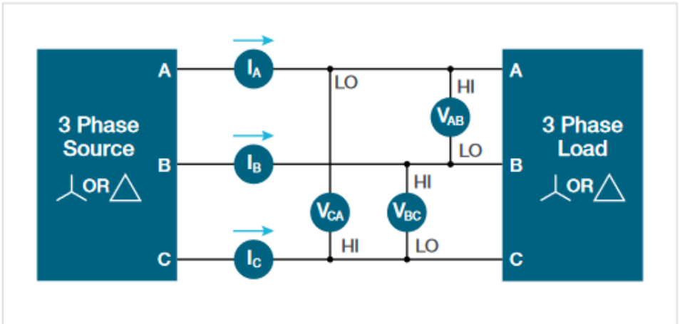
三相三线 (3V3I)
