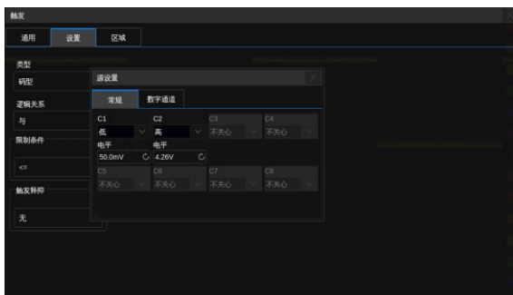
模拟通道的逻辑设置
