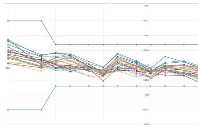
典型值 0.5 % FS的直流增益精度
