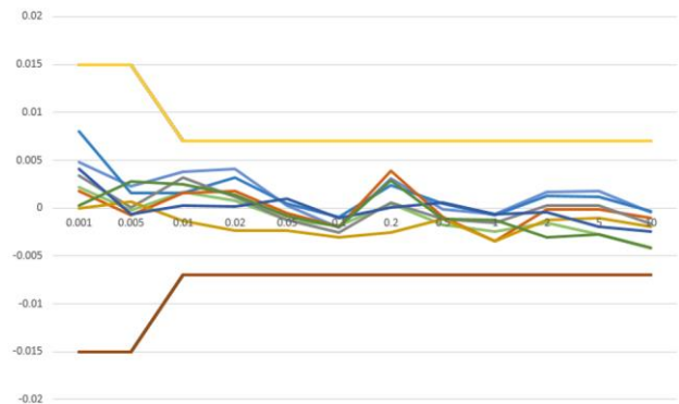
典型值 0.5 % FS 的直流增益精度
